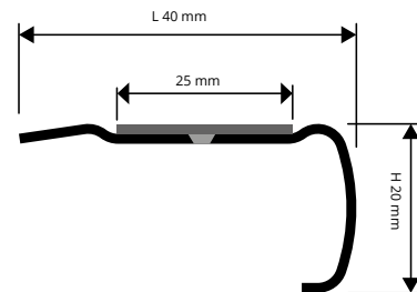
PSYGRACS 4020
